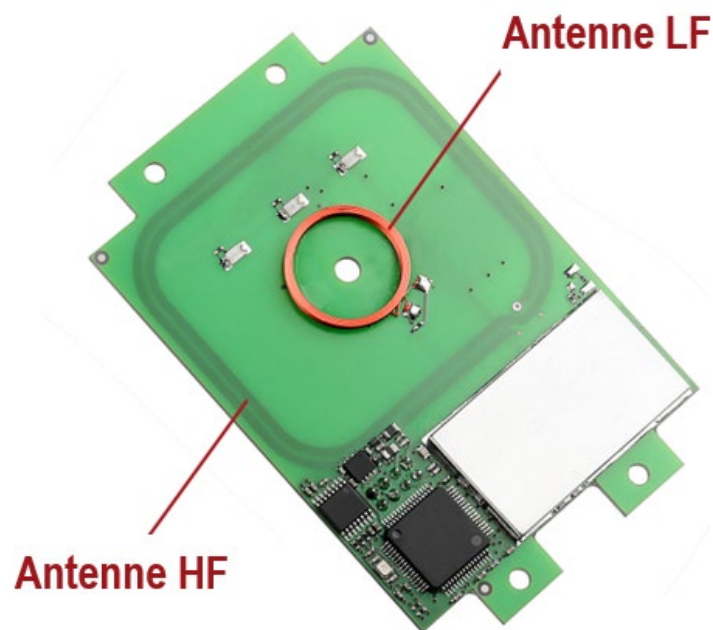
TWN4 MultiTech 2 LEGIC M LF HF (image d'exemple)
