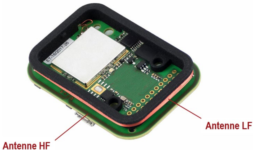
TWN4 MultiTech 3 M BLE
