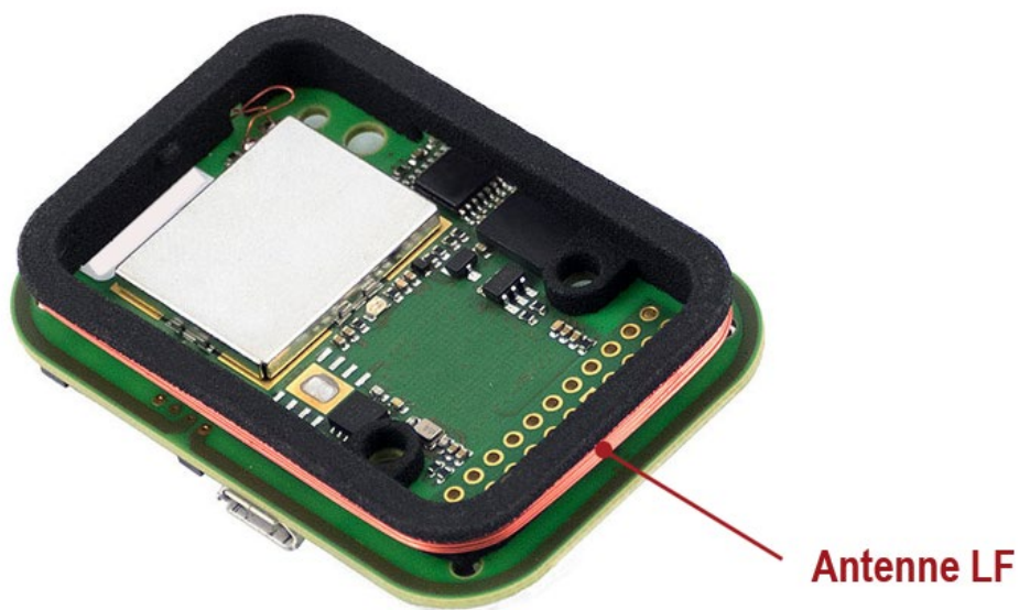
TWN4 MultiTech 3 M LF – Vue du dessous
