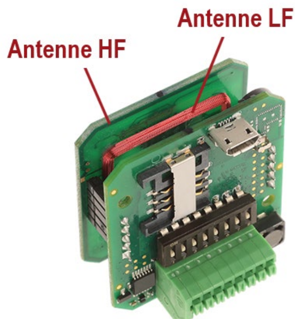
CI contenu dans TWN4 Palon Compact Wall Light
